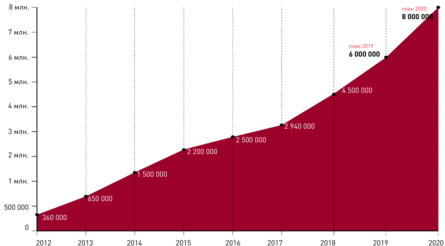
Динамика производства Завода «Форте Пром ГмбХ», шт. секц.
